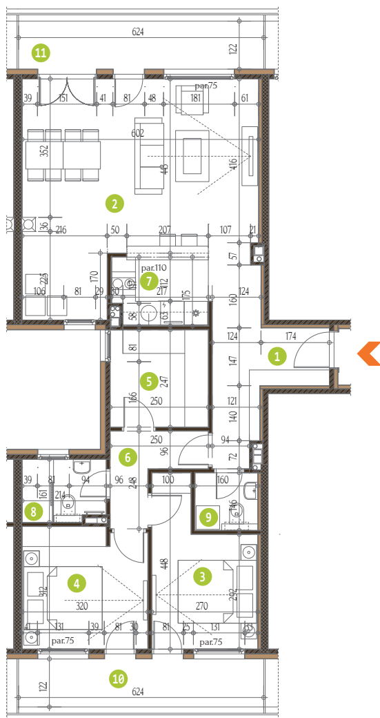
Osnova stana
